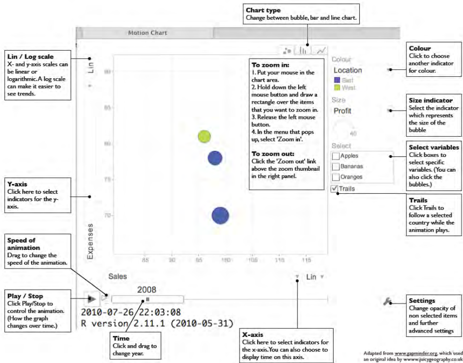
Figure1: Google モーションチャートの概要. plot(gvisMotionChart(Fruits, idvar='Fruit', timevar='Year')) の出力のスクリーンショット.
